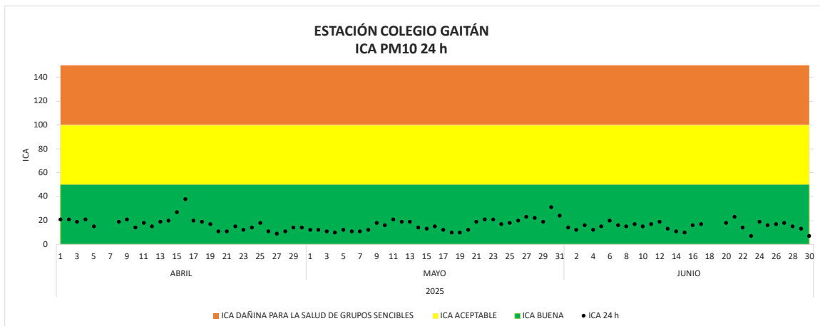
Imagen 39. ICA PM10 24 horas Estación Colegio Gaitán abril a junio de 2025.
