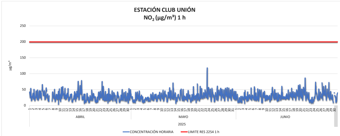
Imagen 24. Concentración NO 2 1 hora Estación Club Unión abril a junio de 2025
