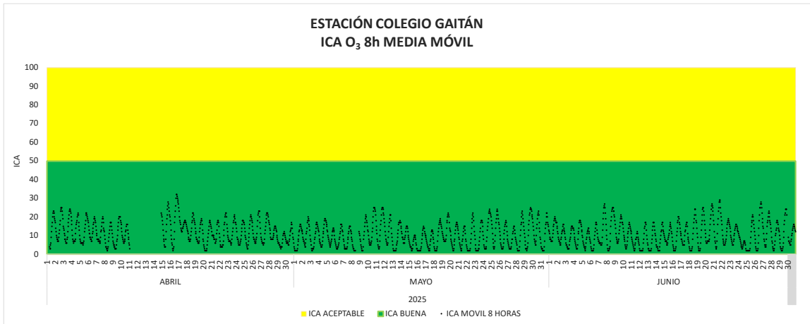
Imagen 47. ICA O 3 8 horas Estación Colegio Gaitán abril a junio de 2025.
