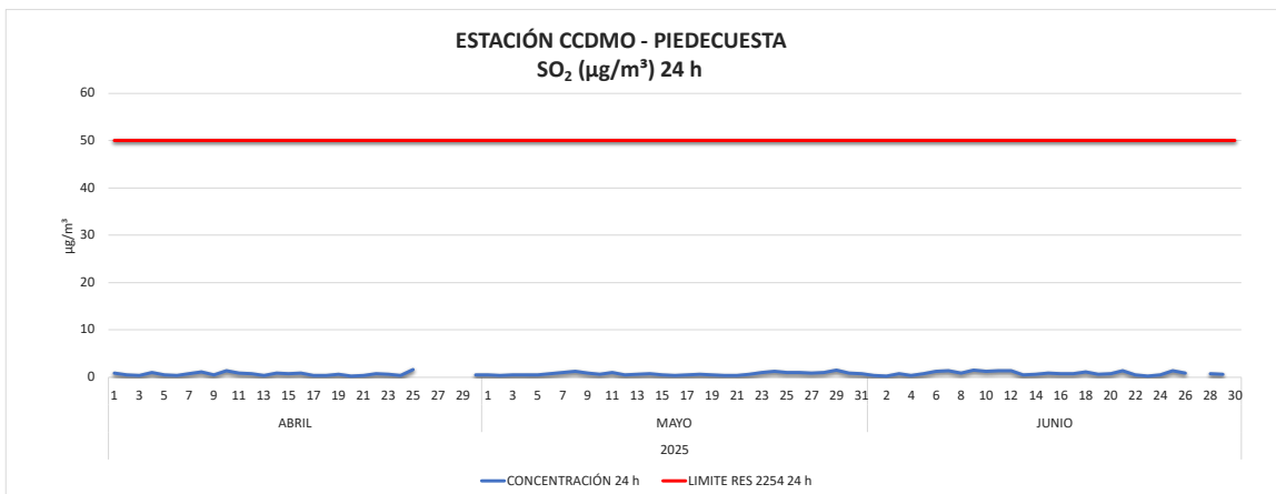
Imagen 29. Concentración SO2 24 horas Estación CCDMO - Piedecuesta abril a junio de 2025.
