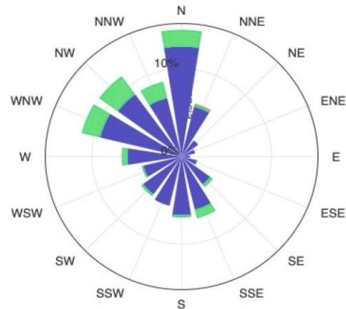
Imagen 69. Rosa de los Vientos Nocturna Estación Colegio Gaitán abril a junio de 2025.
