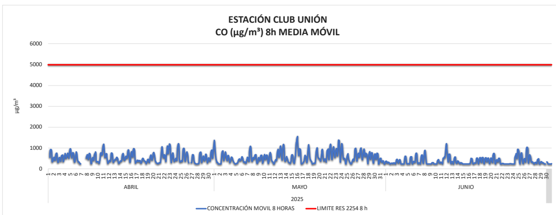
Imagen 31. Concentración CO 8 horas Estación Club Unión abril a junio 2025.
