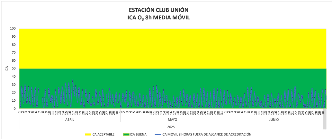
Imagen 46. ICA O 3 8 horas Estación Club Unión abril a junio de 2025
