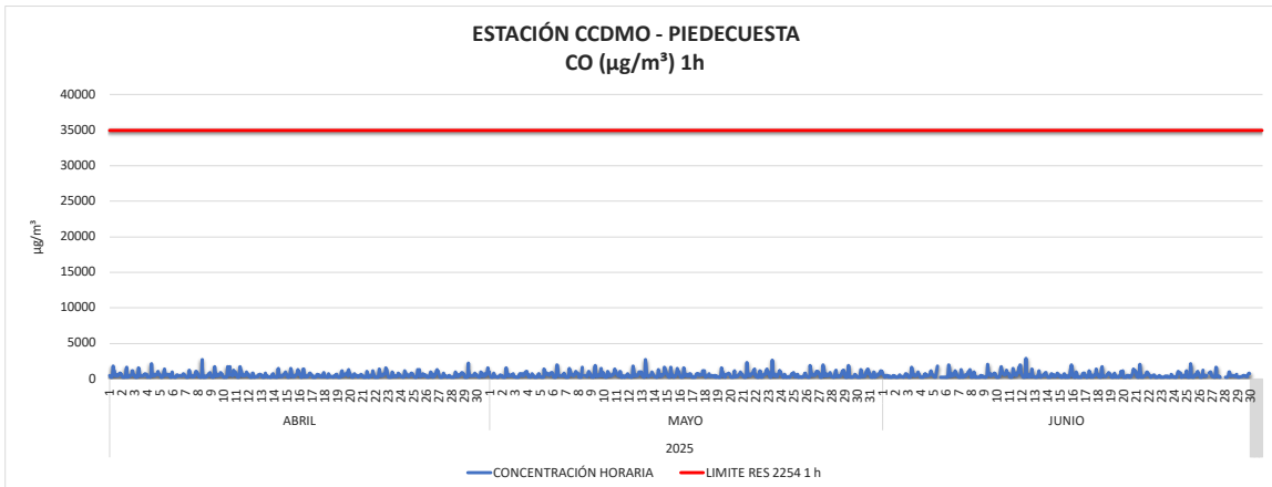
Imagen 32 Concentración CO 1 hora Estación CCDMO - Piedecuesta abril a junio de 2025
