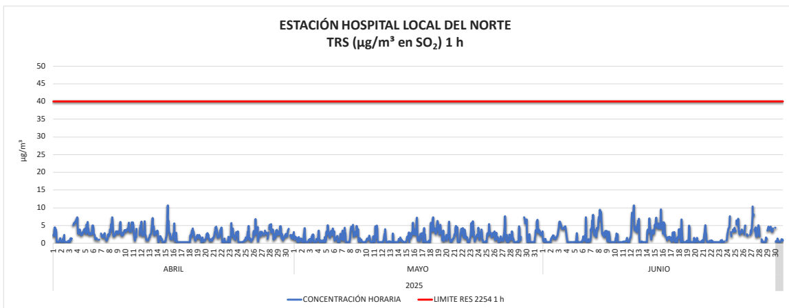
Imagen 34. Concentración TRS 1 hora Estación Hospital Local del Norte abril a junio de 2025.
