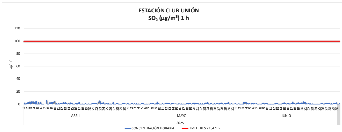
Imagen 26. Concentración SO 2 1 hora Estación Club Unión abril a junio de 2025.
