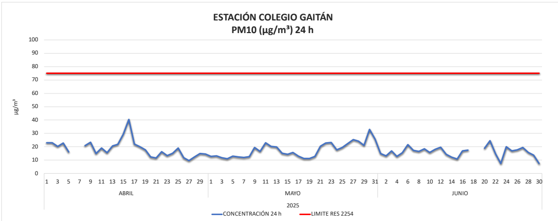
Imagen 13. Concentración PM10 24 horas Colegio Gaitán abril a junio de 2025
