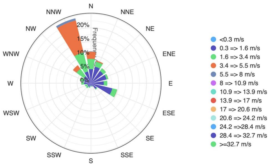
Imagen 70. Rosa de los Vientos Total Estación Hospital Local del Norte abril a junio de 2025.
