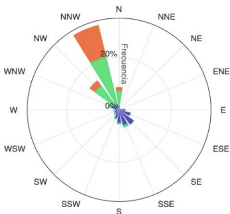
Imagen 65. Rosa de los Vientos Diurna Estación Club Unión abril a junio de 2025.
