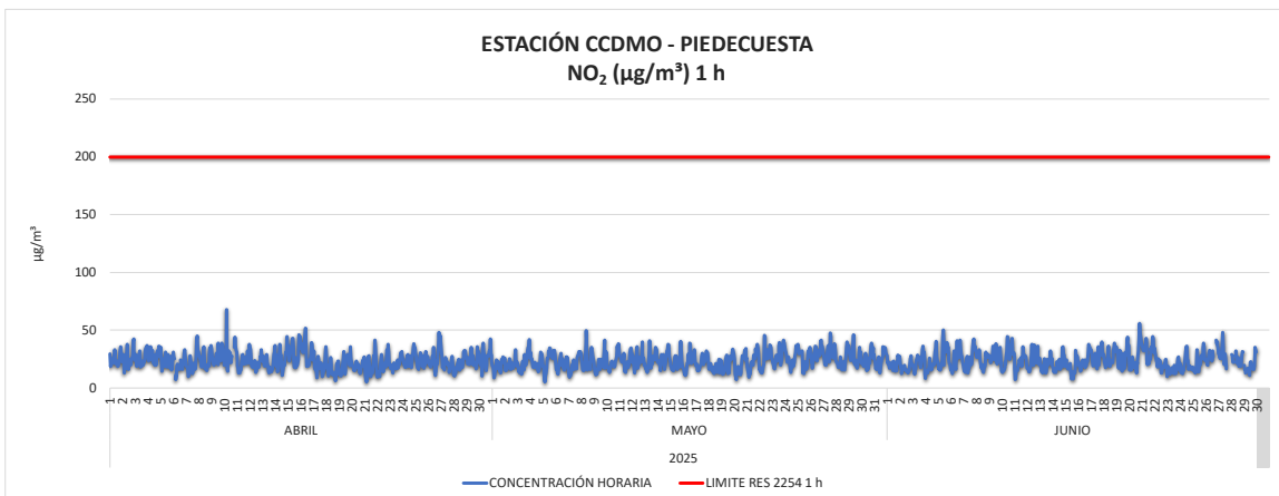
Imagen 25 Concentración NO 2 1 hora Estación CCDMO – Piedecuesta abril a junio de 2025.
