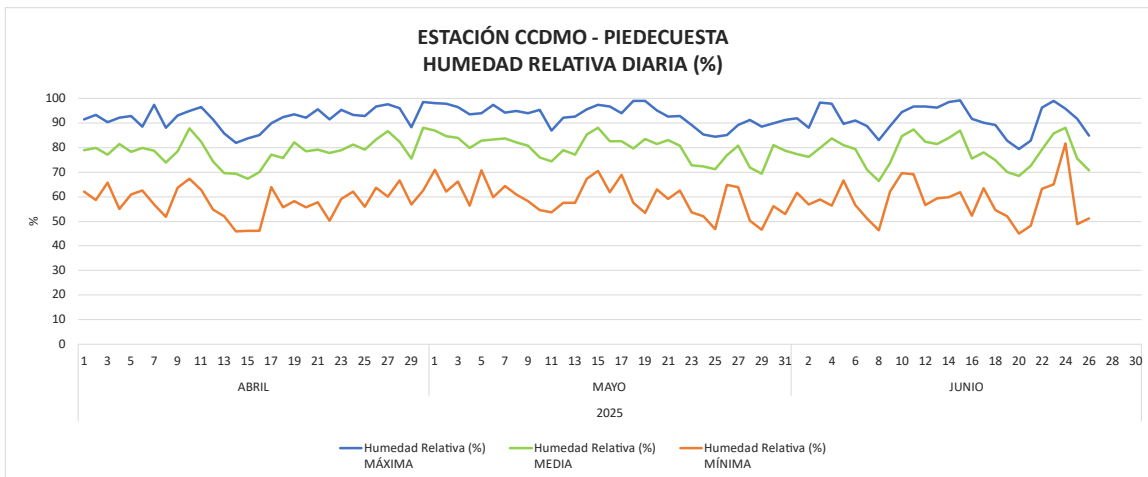
Imagen 79. Humedad Relativa Estación CCDMO - Piedecuesta abril a junio de 2025.
