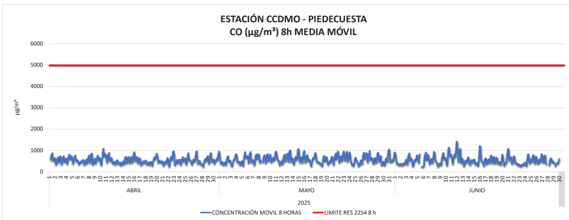
Imagen 33. Concentración CO 8 horas media móvil Estación CCDMO - Piedecuesta abril a junio de 2025
