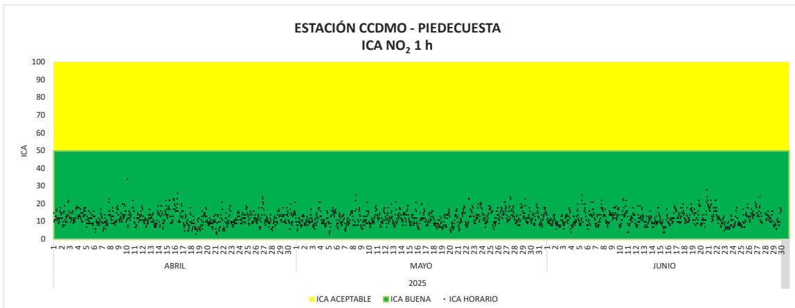
Imagen 51. ICA NO2 1 hora Estación CCDMO- Piedecuesta abril a junio de 2025.
