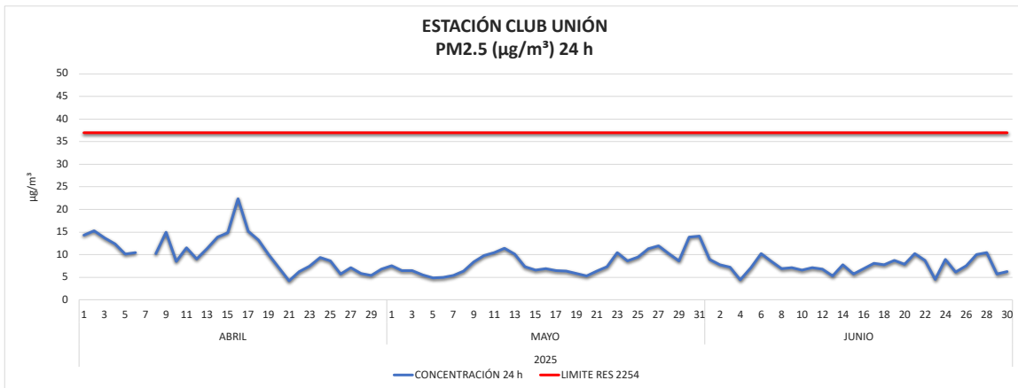
Imagen 16. Concentración PM 2.5 24 horas Estación Club Unión abril a junio de 2025.
