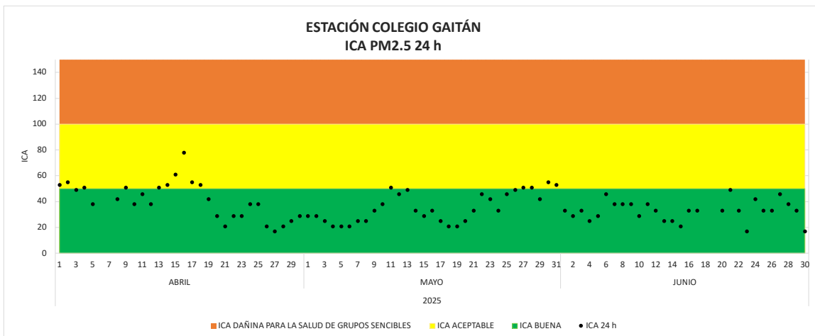
Imagen 43. ICA PM2.5 24 horas Colegio Gaitán abril a junio de 2025
