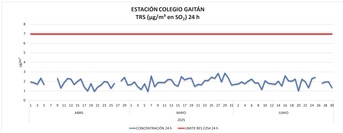
Imagen 37. Concentración TRS 24 horas Estación Colegio Gaitán abril a junio de 2025.
