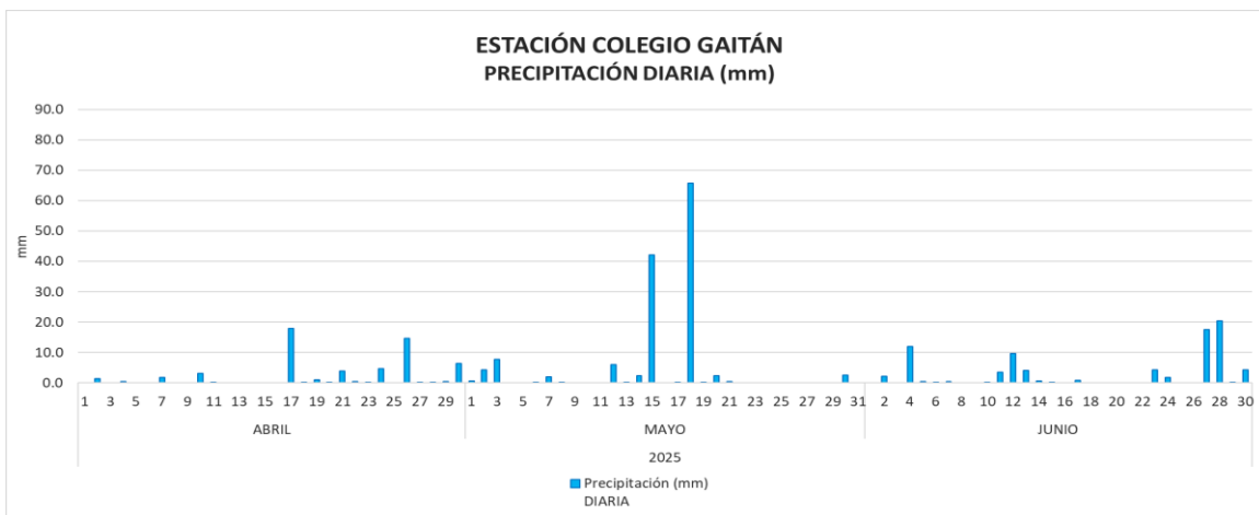
Imagen 61. Precipitación Horaria Estación Colegio Gaitán abril a junio de 2025.
